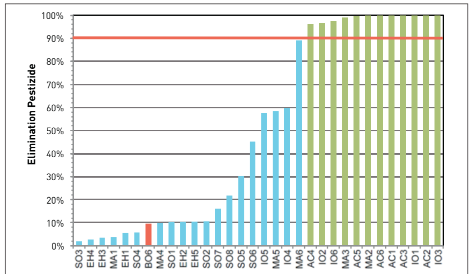
Abb. 2: Mittlere Elimination der Pestizide in den Batchversuchen.
