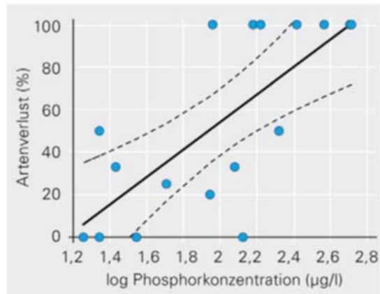
Abbildung 2: Zusammenhang von maximaler Phosphorkonzentration und Verlust von endemischen Felchenarten. Je höher die maximale Konzentration, desto grösser der Artenverlust bei den Felchen. Diese, und andere Arbeiten illustrieren, dass die heute oligotrophen Seen zahlreiche Endemiten beherbergen (Quelle: Vonlanthen et al., 2012)
