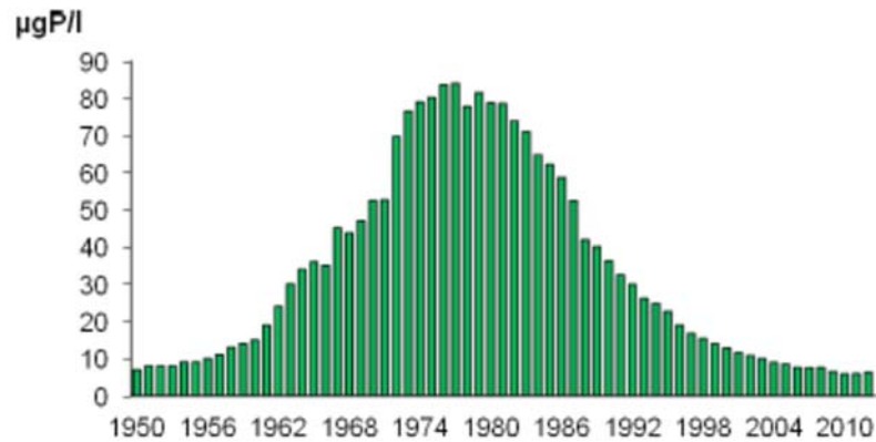
Abbildung 1: Gesamt-P Jahresmittelwerte in Bodensee-Obersee von 1950 bis 2012. (Quelle: Internationale Gewässerschutzkommission für den Bodensee IGKB 2013)
